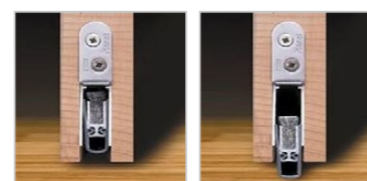
AJTÓLAP ALJÁBA ÉPÍTETT AUTOMATA KÜSZÖB NYITOTT ÉS ZÁRT ÁLLAPOTBAN az ajtólap aljába beépíthető szerkezet az ajtólap nyitott vagy zárt állapotával összhangban emelkedik fel, vagy süllyed a padlóra
